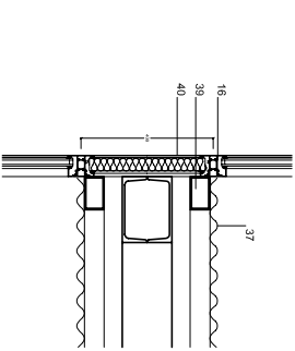
Plan / Planta
